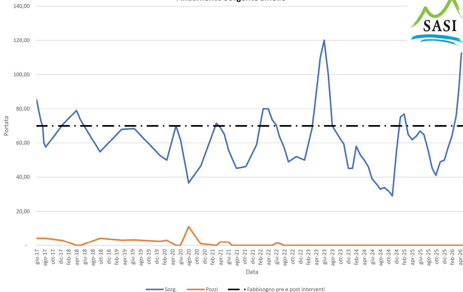
Andamento Sorgente Sinello
