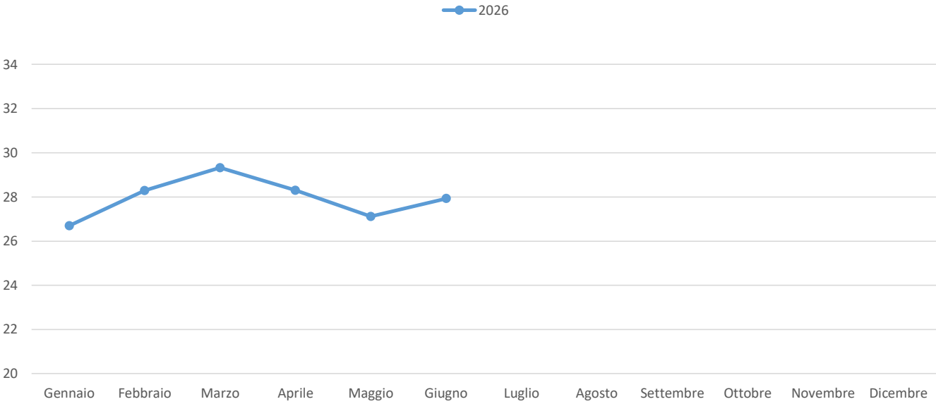
PORTATE MEDIE ADDOTTE/CAPTATE in l/s Pozzo Monte Cervaro
