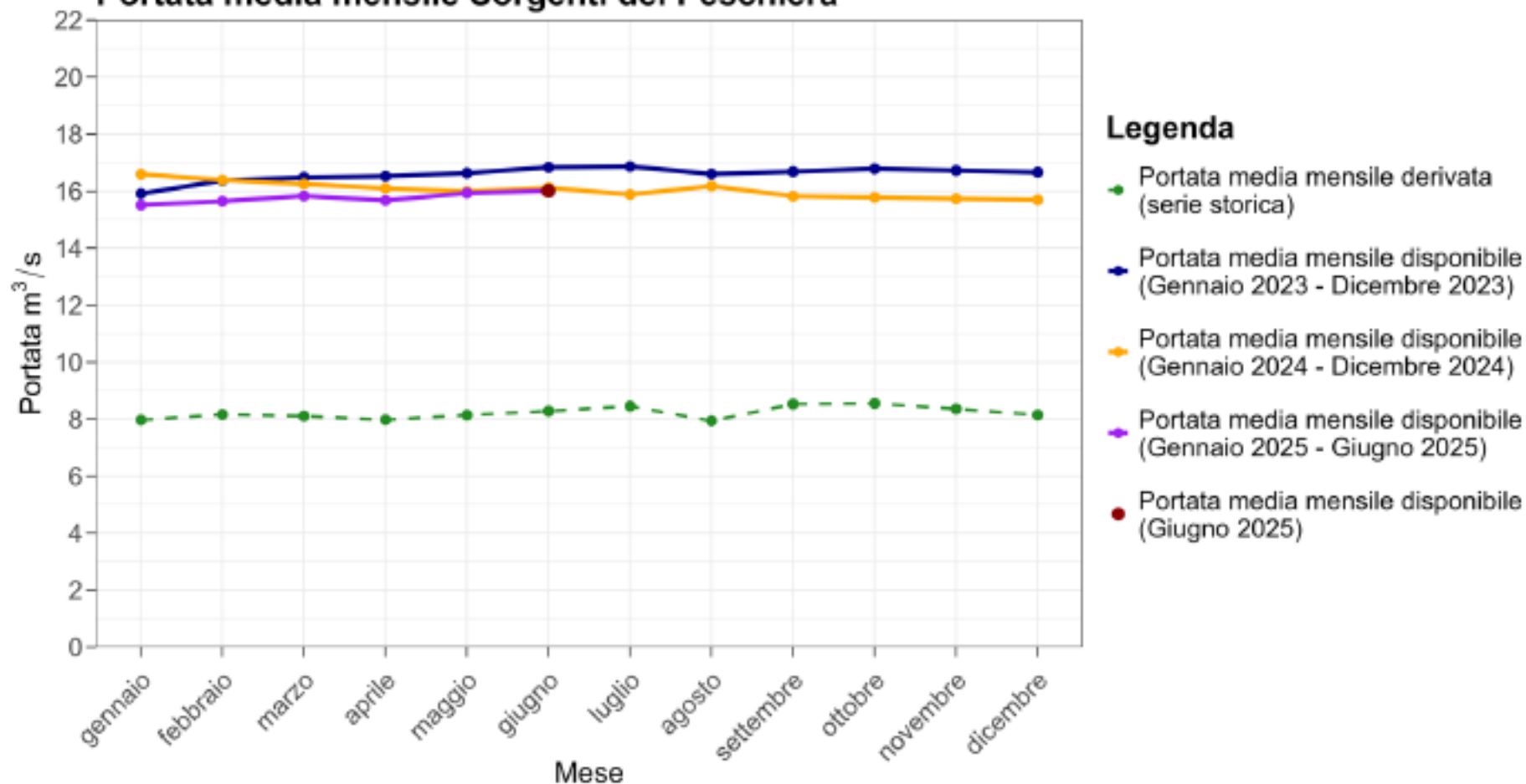
Figura 5. Andamento delle portate medie mensili totalizzate dal sistema di sorgenti del Peschiera
