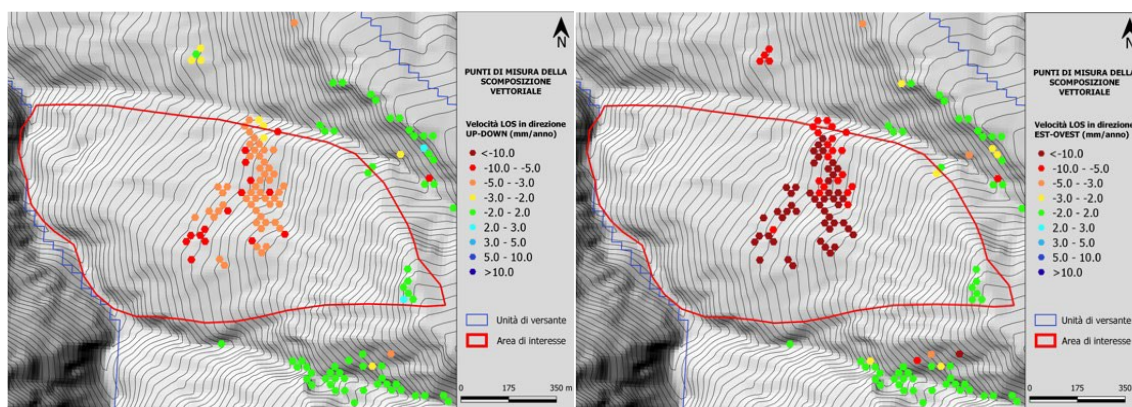
Risultato della scomposizione vettoriale per la frana in località Fano Adriano (Abruzzo). Nel pannello di sinistra vengono mostrati i movimenti lungo la direzione verticale, mentre a destra lungo quella orizzontale
