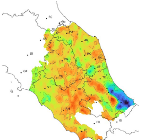
SPEI a 6 mesi relativo al 30 aprile 2025
