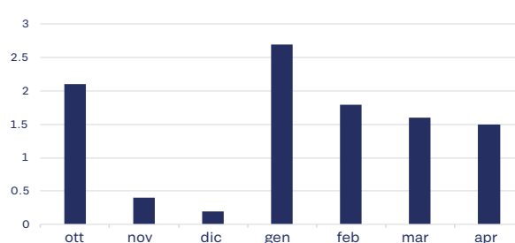
Umbria - Scostamento temperatura media rispetto al 1991-2020 (°C)
