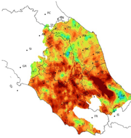
SPI a 24 mesi relativo al 30 aprile 2025
