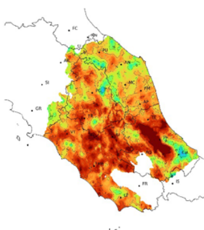
SPEI a 24 mesi relativo al 30 aprile 2025
