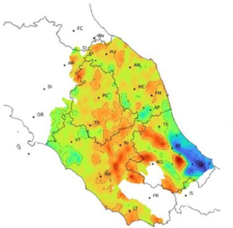
SPI a 6 mesi relativo al 30 aprile 2025
