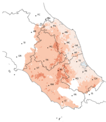
Marzo 2025 - Scostamento temperatura media mensile rispetto a 1991-2020
