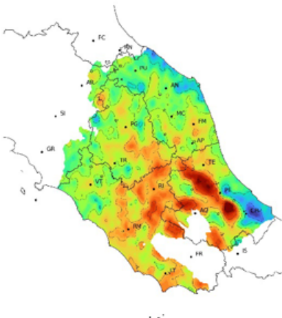
SPI a 12 mesi relativo al 30 aprile 2025
