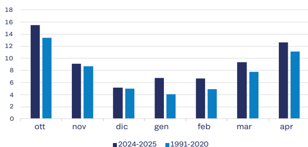
Umbria - Temperatura media (°C)
