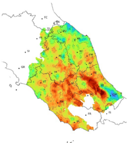
SPEI a 12 mesi relativo al 30 aprile 2025
