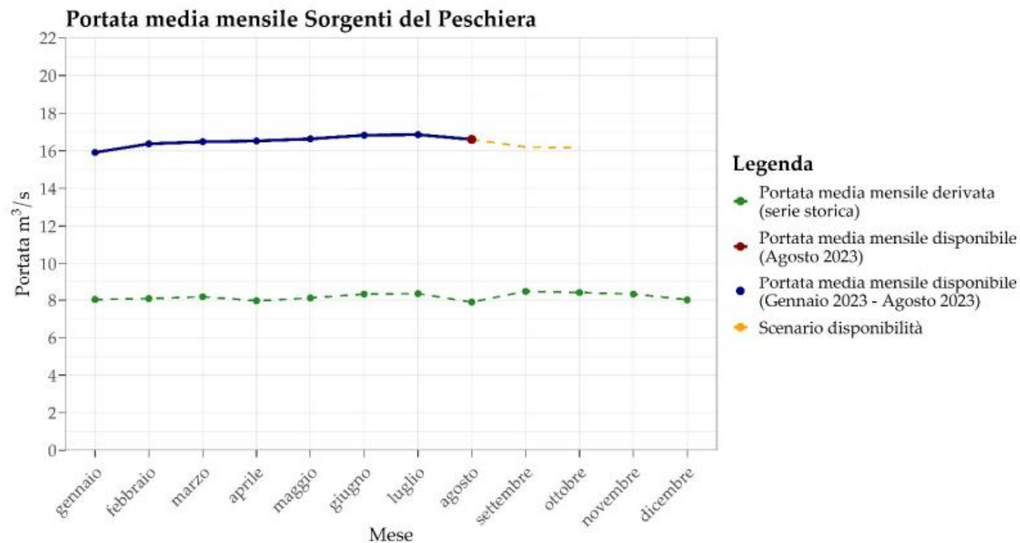
Figura 4. Andamento delle portate medie mensili totalizzate dal sistema di sorgenti del Peschiera
